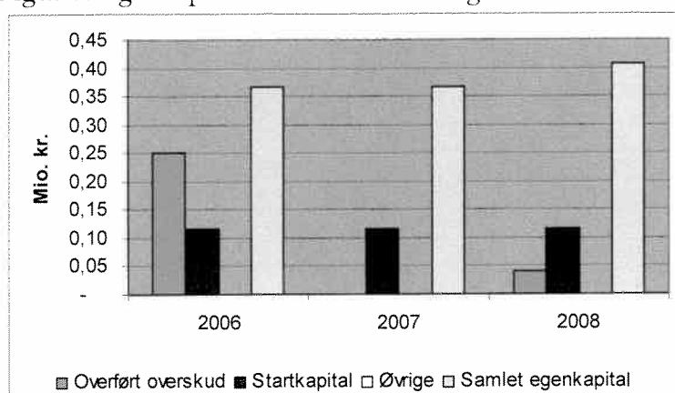
Figur 3: Egenkapitalens sammensætning
