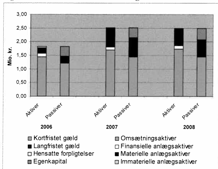
Figur 2: Balancens sammensætning
